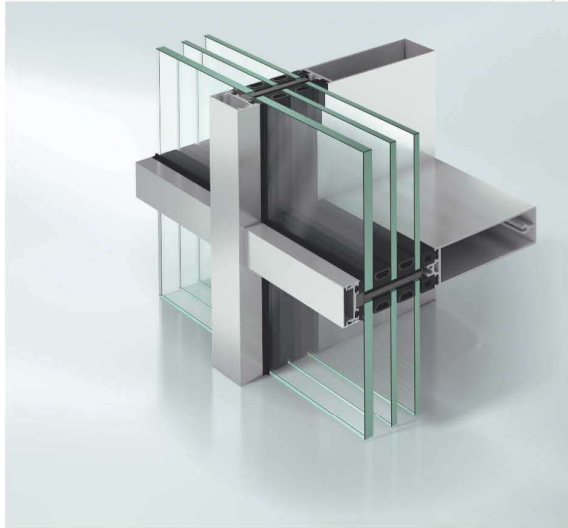
Schüco Façade FWS 35 PD.SI
